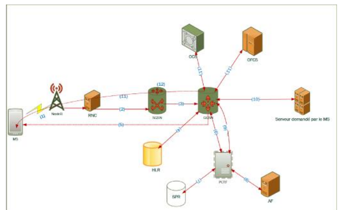
Fig.6 Principe de la facturation dans un réseau numérique d'opérateur
